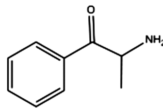
(b) Catinona
